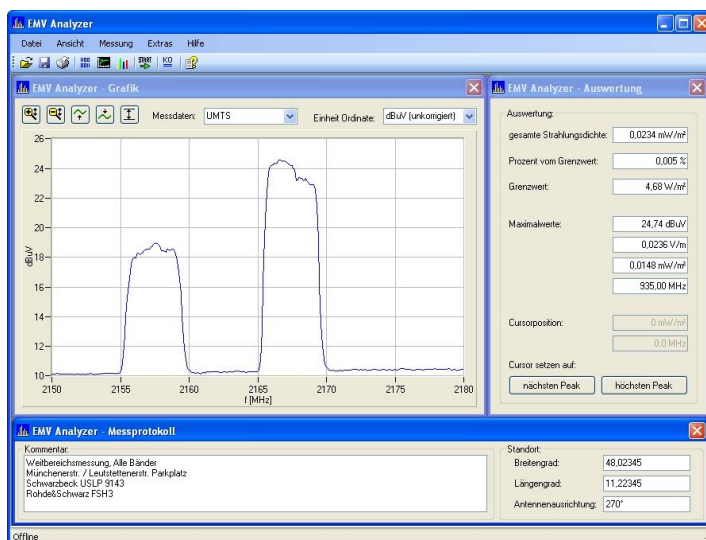
EMV-Analyser zur Messung der Strahlungsdichte mit R&S Spektrumsanalysator
